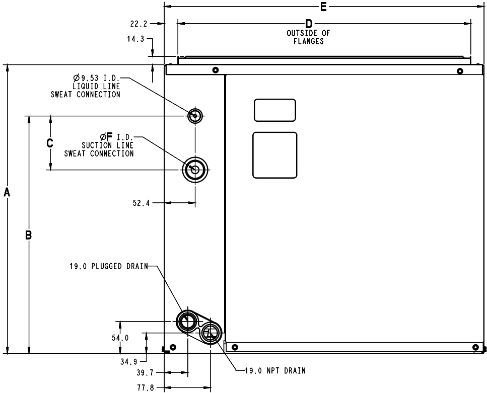
Fig. 3 – Dimensions (Metric)
