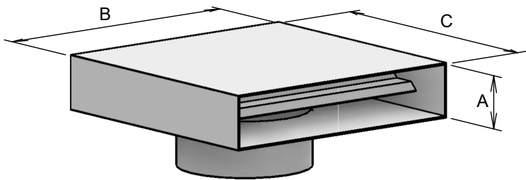
TOESPACE HEAD
