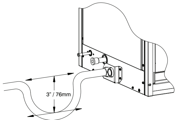
Fig. 8 – Condensate Trap
